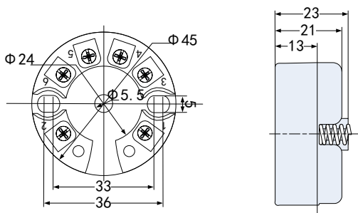
图2.1 温度模块尺寸（单位：mm）
