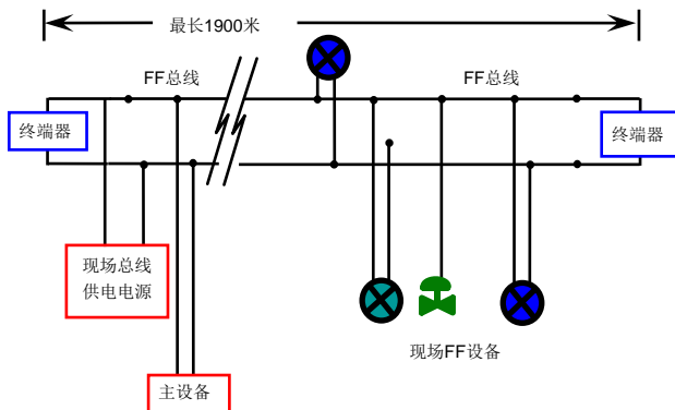
图3.2 FF 总线连接
