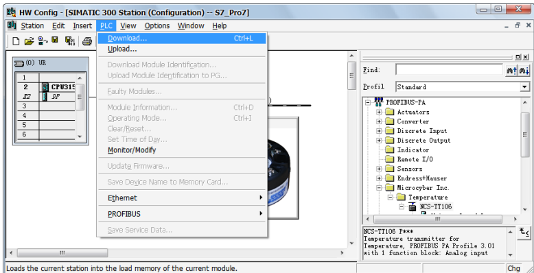
图4.7 下载组态信息到 PLC
