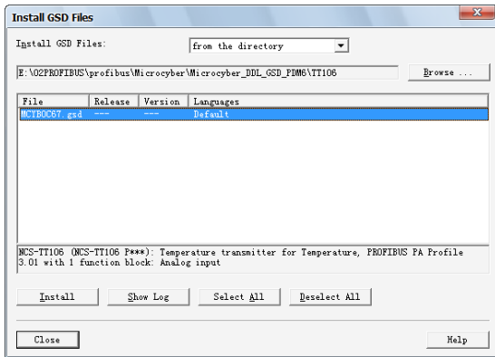
图4.5 安装 GSD 文件
