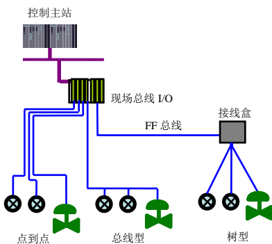
图3.1 FF 网络拓扑
