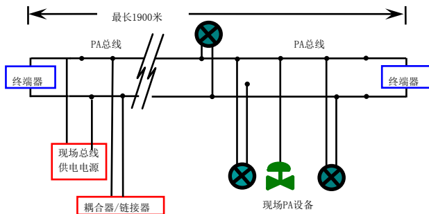
图4.2 PROFIBUS PA 总线连接
