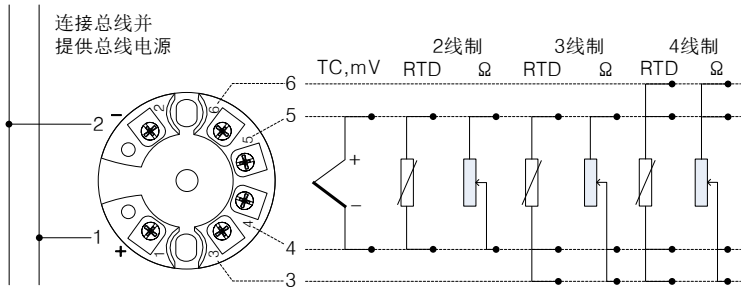
图2.3 温度模块接线示意图
