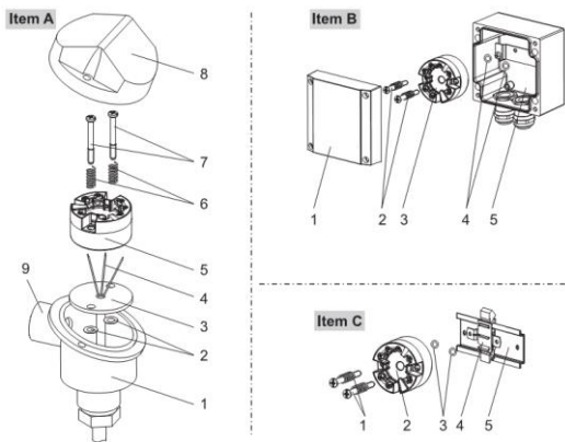
图2.2 温度模块安装示意图
