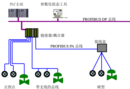
图4.1 PROFIBUS PA 网络拓扑
